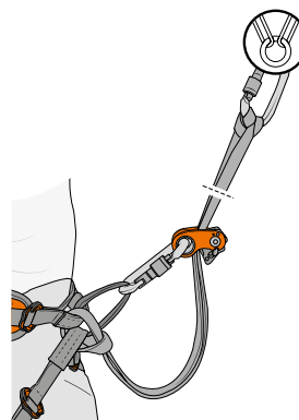
4 Positioning adjustment on webbing Ajuste de posición en cinta
